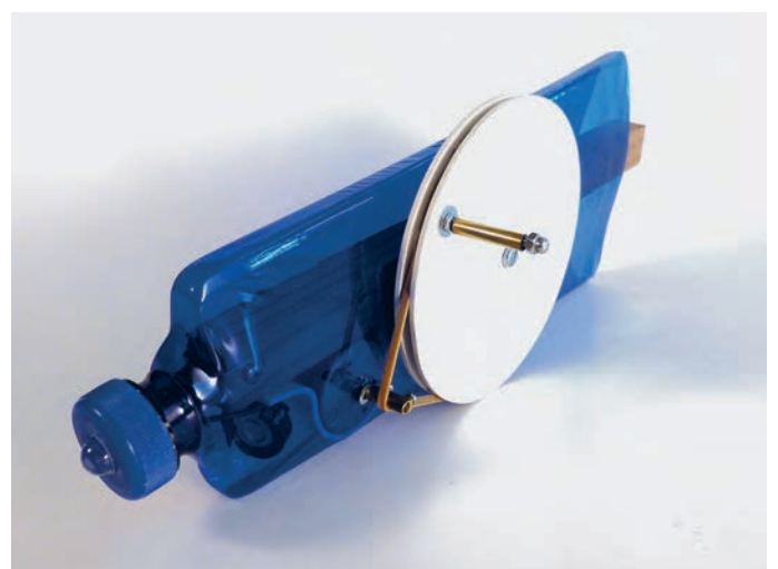
Die Taschenlampen im Recyclingobjekt nutzen einen Elektrolyt-Kondensator als Speicher – dessen sofortige Entladung wird durch eine zusätzliche Diode verhindert.
